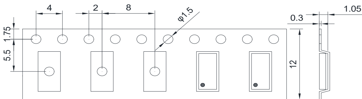
Fig.4 编带包装示意图。
