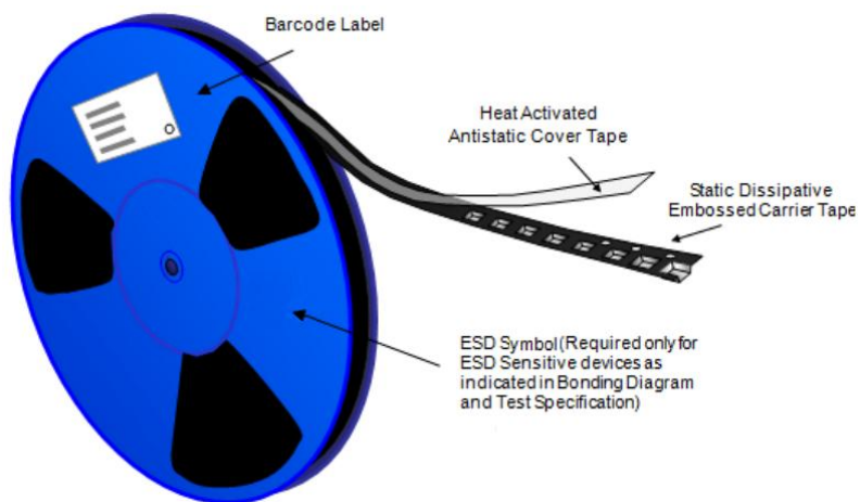
Fig.4 编带包装示意图。
