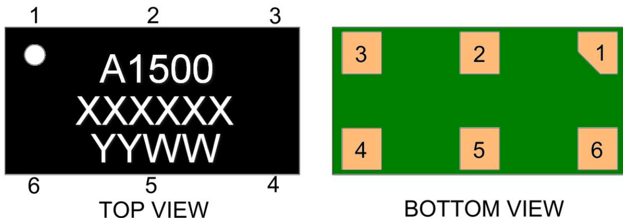
Fig.1 A-1500-075 传感器的位置和外形封装图（单位：mm）。
