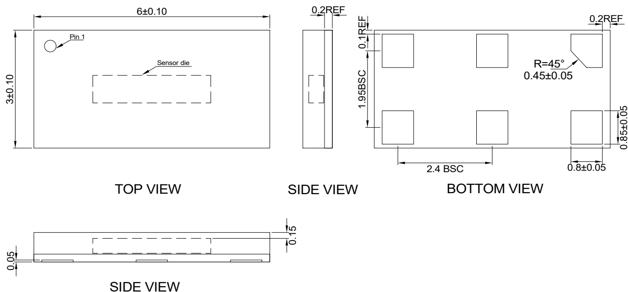
Fig.1 A-1500-075 传感器的位置和外形封装图（单位：mm）。
