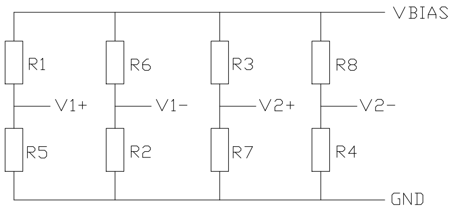
Fig.2 A-1500-075 传感器的脚位定义和内部原理图。
