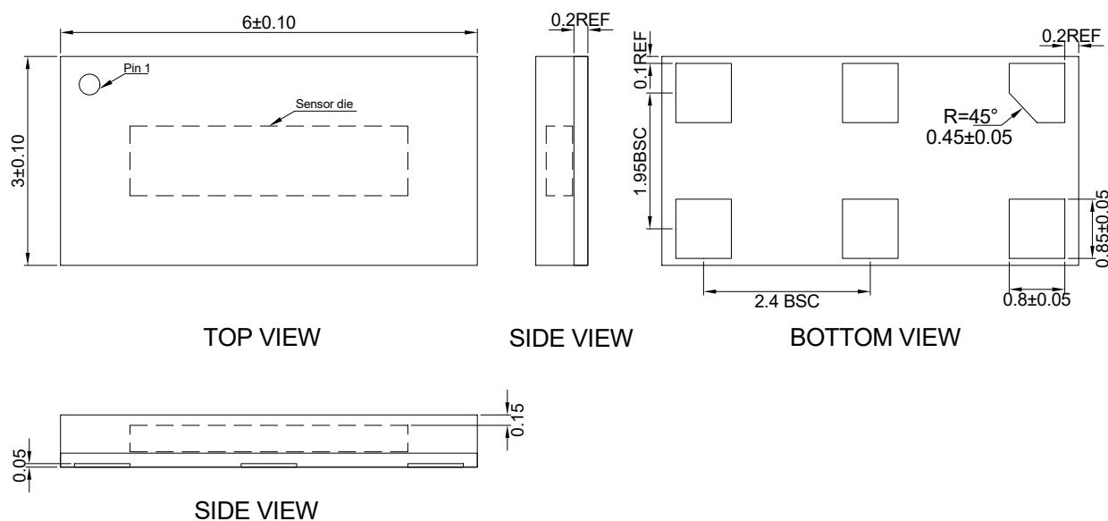
Fig.1 A-2000-075 传感器的位置和外形封装图（单位：mm）。
