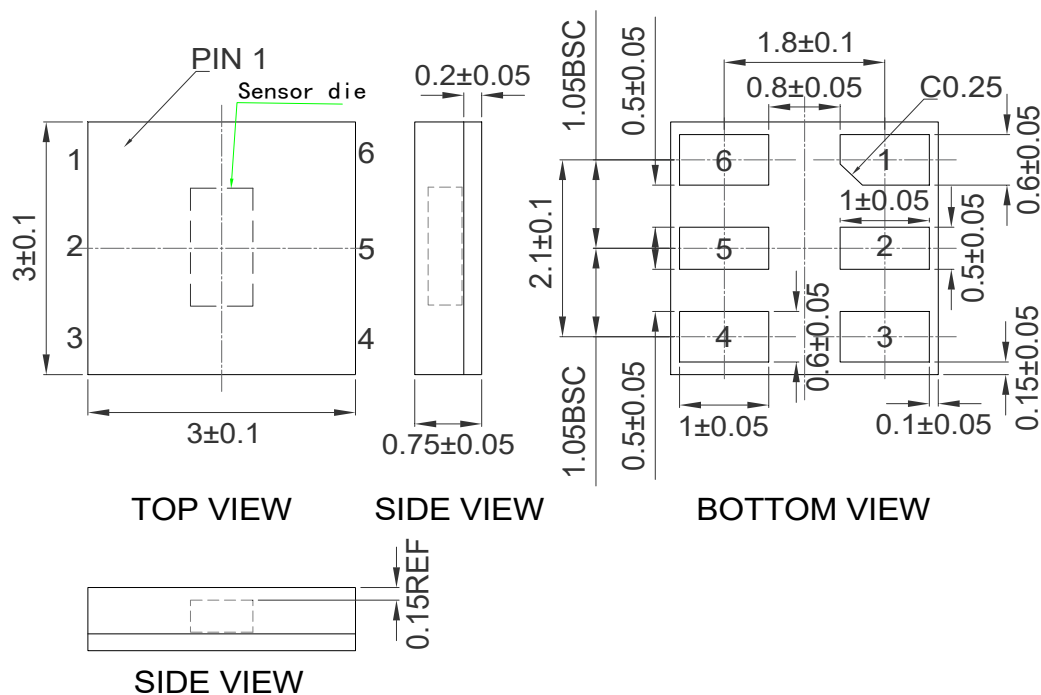
Fig.1 A-0625-075 传感器的位置和外形封装图（单位：mm）。
