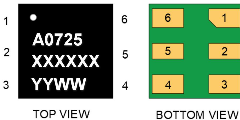
Fig.1 A-0725-075 传感器的位置和外形封装图 (单位: mm)。
