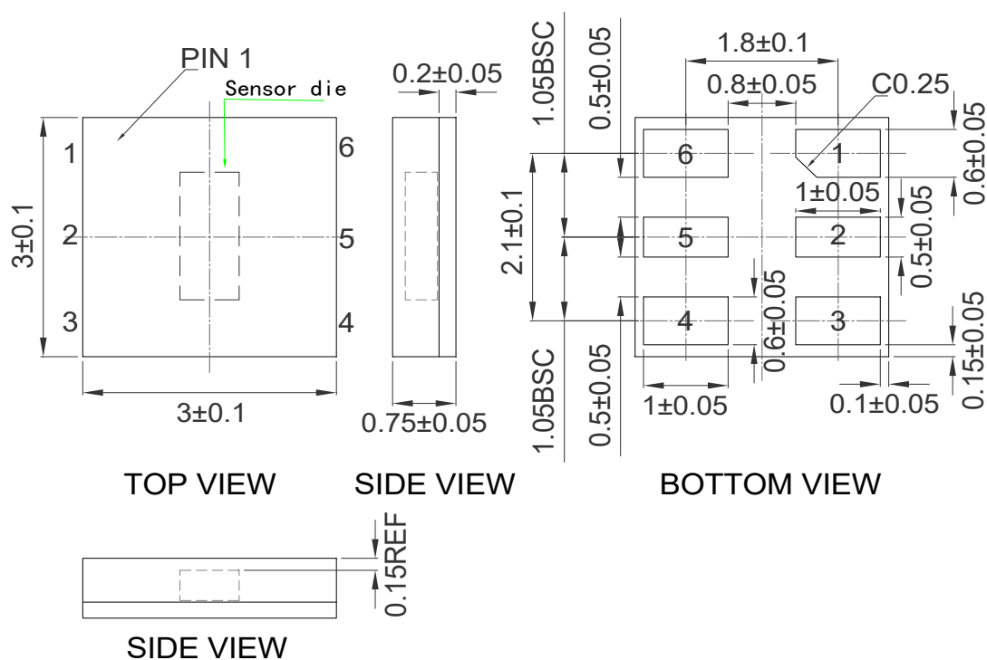
Fig.1 A-0725-075 传感器的位置和外形封装图 (单位: mm)。
