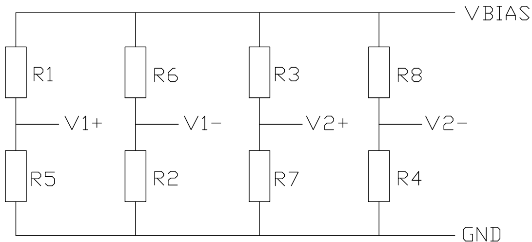
Fig.2 A-0725-075 传感器的脚位定义和内部原理图。
