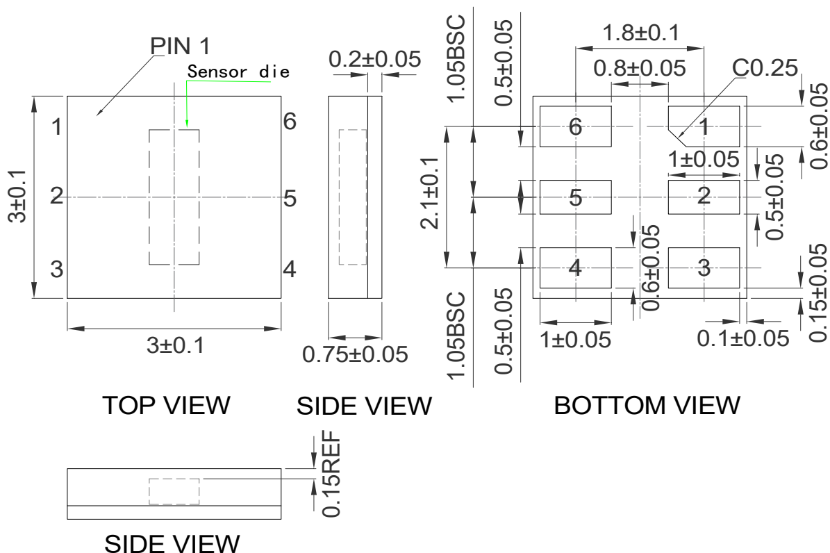
Fig.1 A-0925-075 传感器的位置和外形封装图 (单位: mm)。
