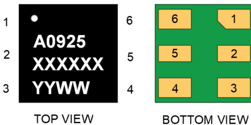
Fig.1 A-0925-075 传感器的位置和外形封装图 (单位: mm)。
