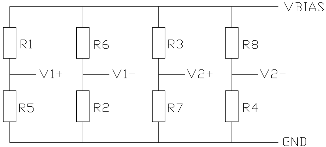
Fig.2 A-0925-075 传感器的脚位定义和内部原理图。
