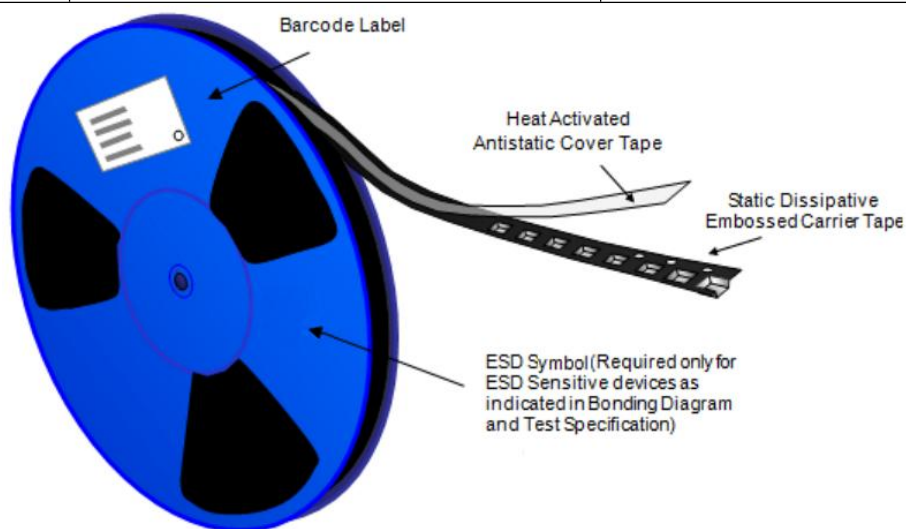
Fig.3 编带包装示意图。
