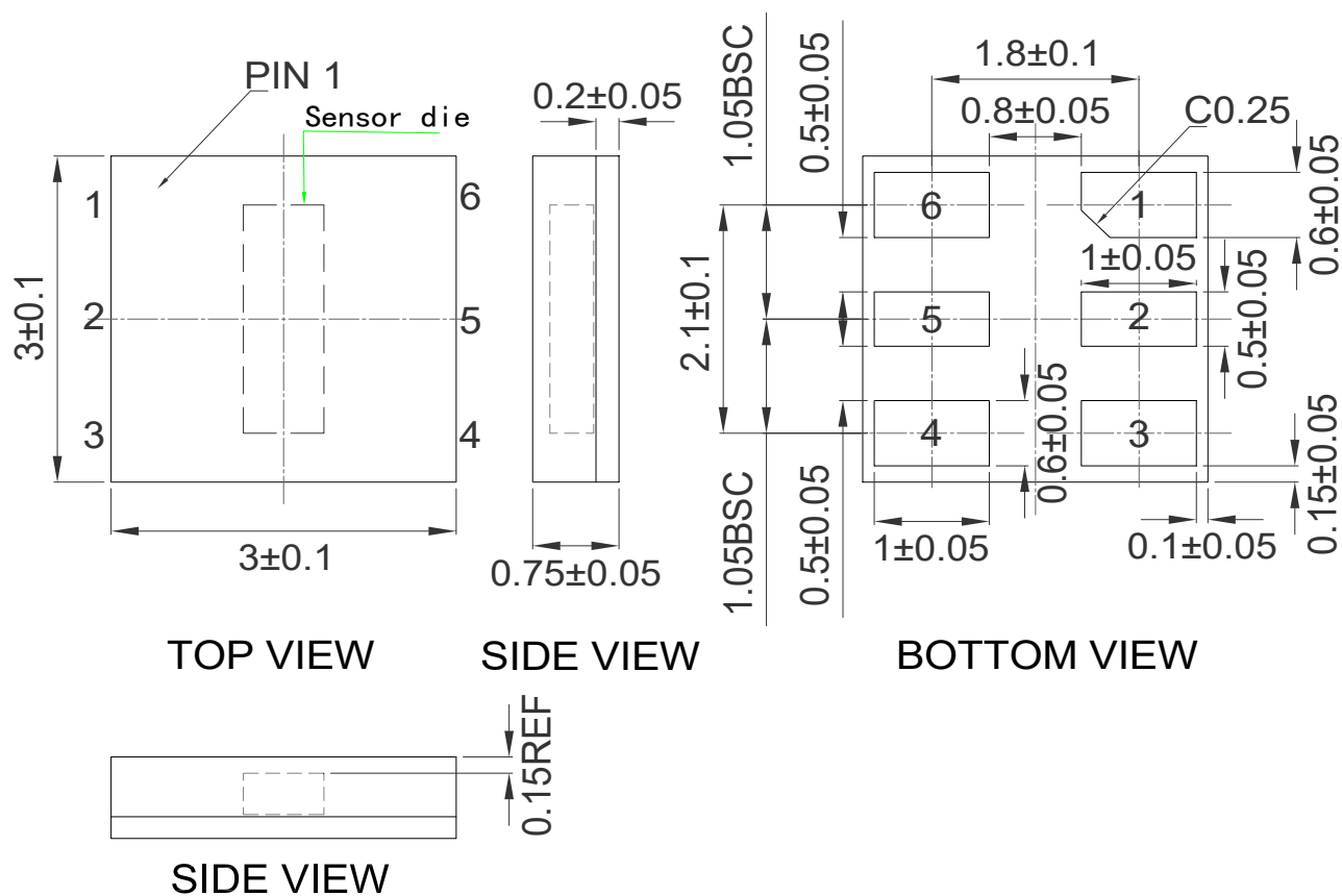
Fig.1 A-1000-075 传感器的位置和外形封装图 (单位: mm)。
