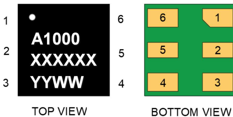
Fig.1 A-1000-075 传感器的位置和外形封装图 (单位: mm)。
